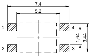
Scale - 5:1
